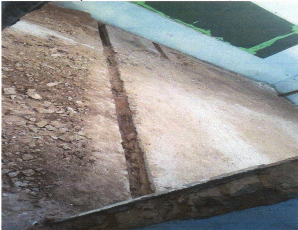
FOTO 04 – ESCAVAÇÃO MANUAL DE VALA PARA VIGA BALDRAME (INCLUINDO ESCAVAÇÃO PARA COLOCAÇÃO DE FÔRMAS). AF_06/2017
