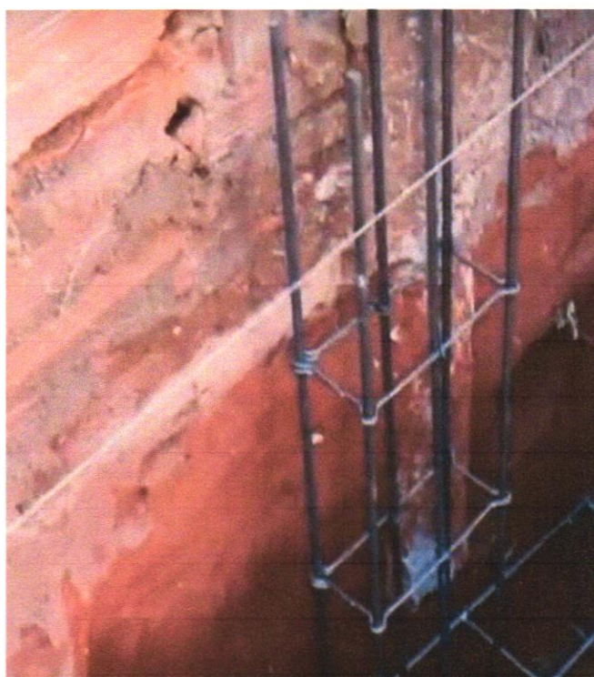
FOTO 14 - Escavação manual para bloco de coroamento ou sapata (sem escavação para colocação de fôrmas). af_06/2017
